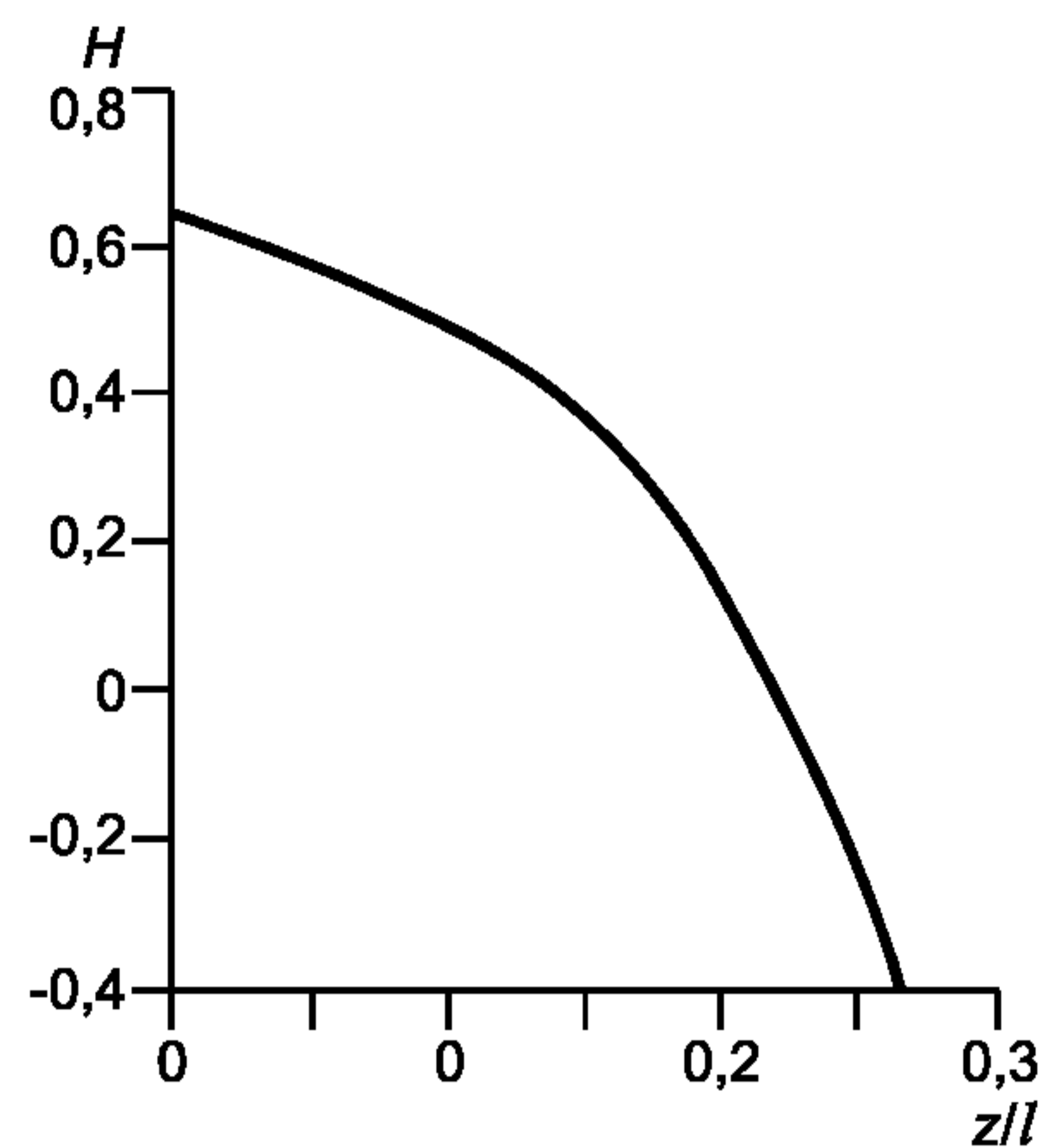
Рисунок В.1 — График для определения коэффициента H
