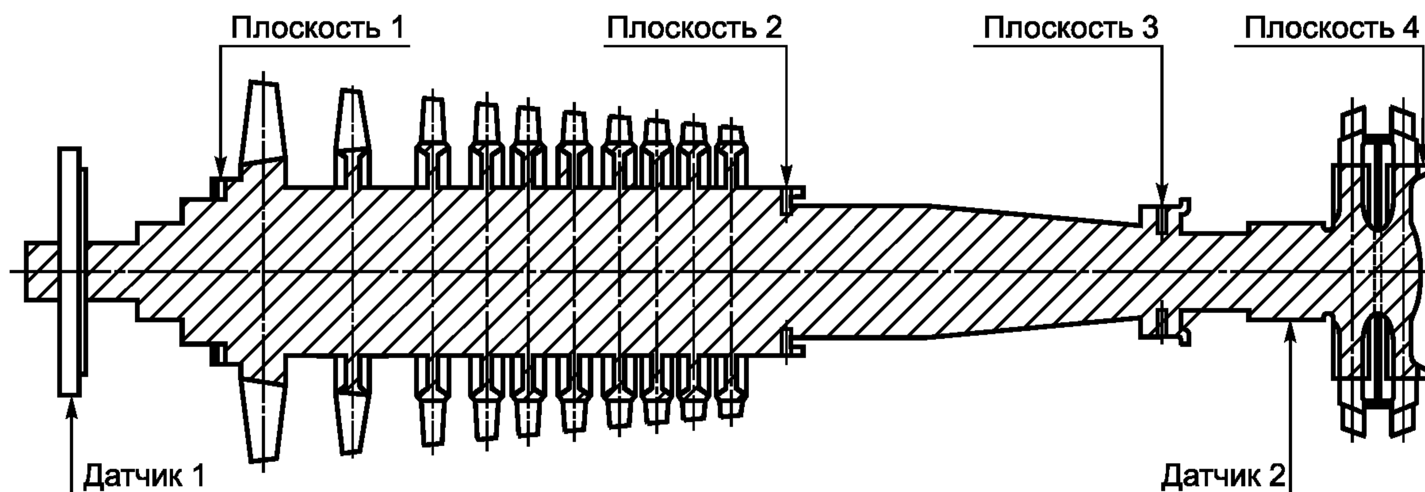
Рисунок D.1 — Ротор турбины
